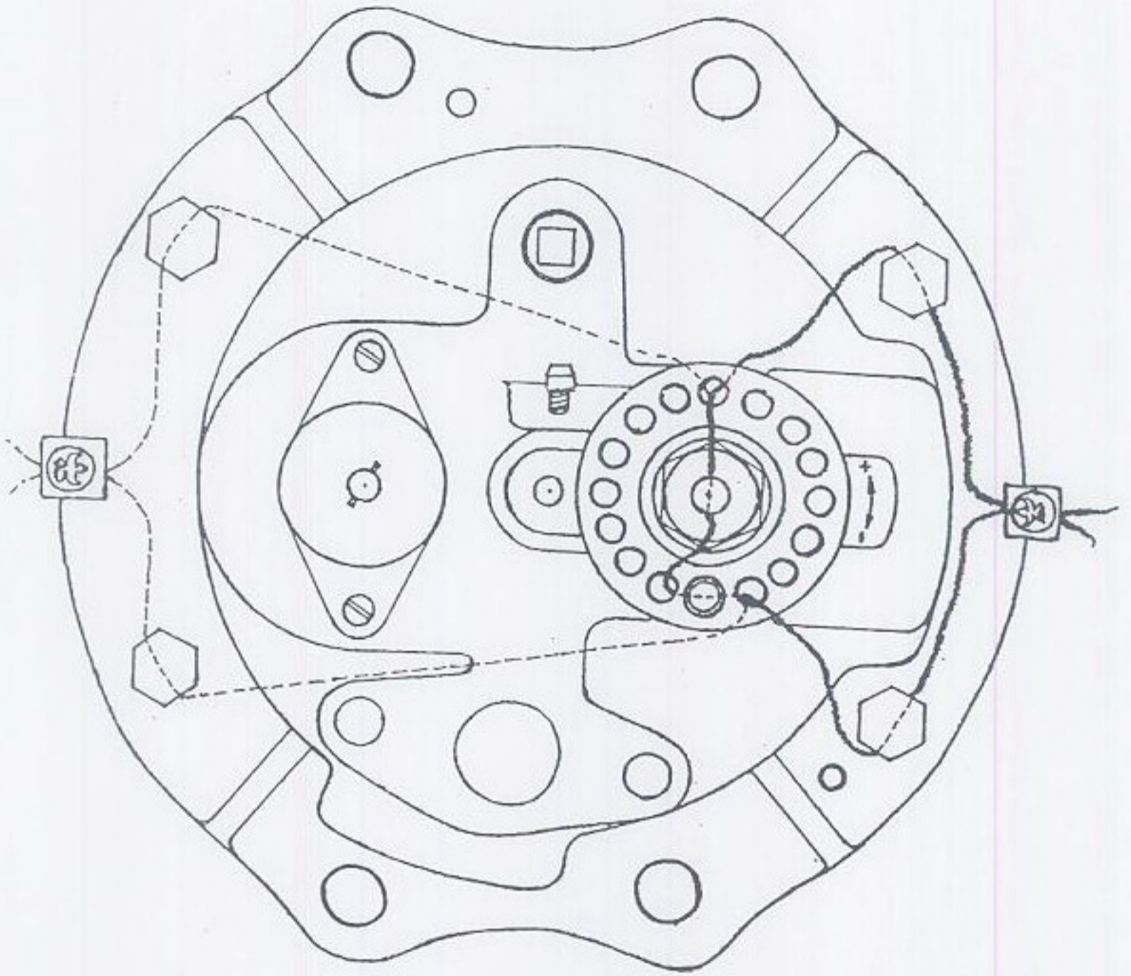
ภาพเครื่อง TOKHEIM มองจากด้านบน การผูกมัดลวดประทับตรา ให้เลือกผูกเพียง ด้านเดียวเท่านั้น โดยให้เห็นเครื่องหมาย คำรับรองอย่างชัดเจน ไม่มีสิ่งใดมาปิดบัง
